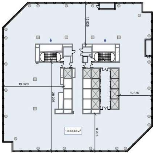
План типового этажа
